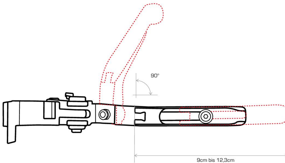
Bremshebel
